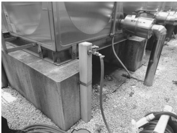
図7 高齢者向け施設において受水槽に蛇口を取り付けた例
