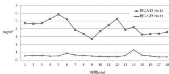
図一七 現場適用結果（吹付時、送風量1330m 3 /min、排気量2000m 3 /min）
