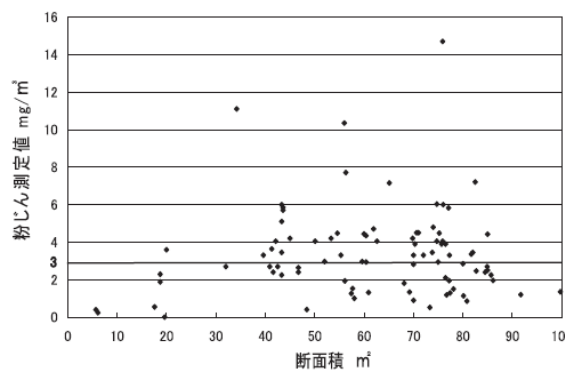
「ガイドライン」後 2005年日本建設機械化協会データ
