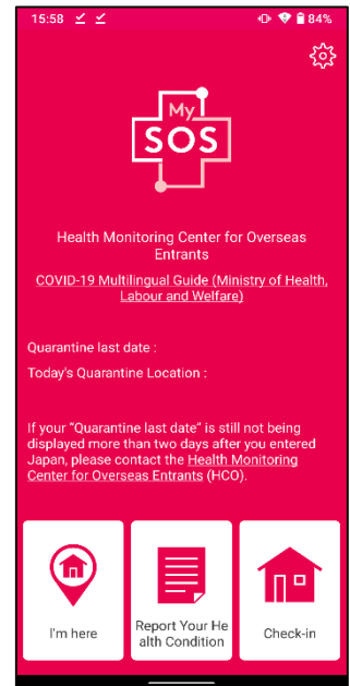
完成注册
