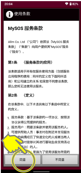
点击“同意”
