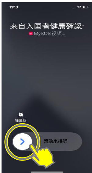
滑动“>”接听
