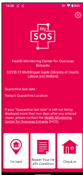
完成注册
