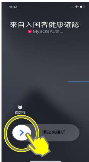
滑动“>”接听
