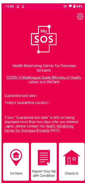
完成注册
