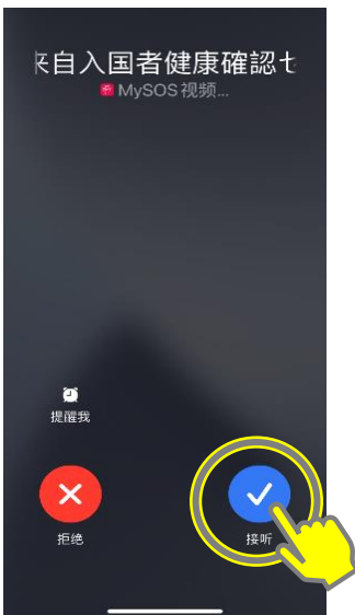
点击接听✓
