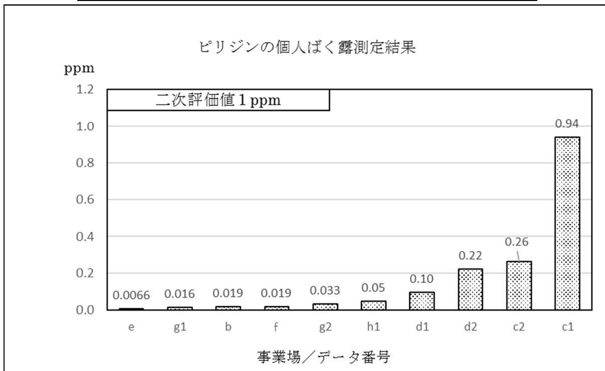
図2 ピリジンの個人ばく露測定結果（追加調査結果を含む。）
