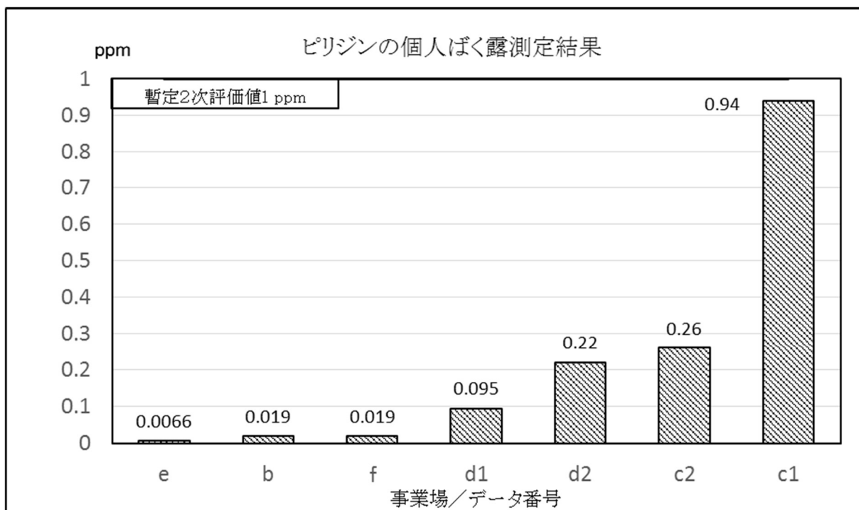
251 図1 ピリジンの個人ばく露測定結果
