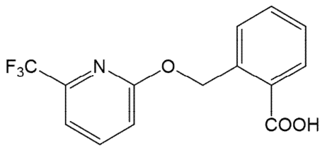
代謝物F
