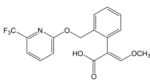
代謝物C
