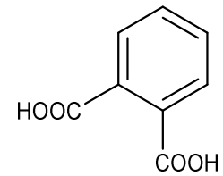
代謝物Z
