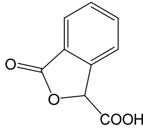
代謝物Y
