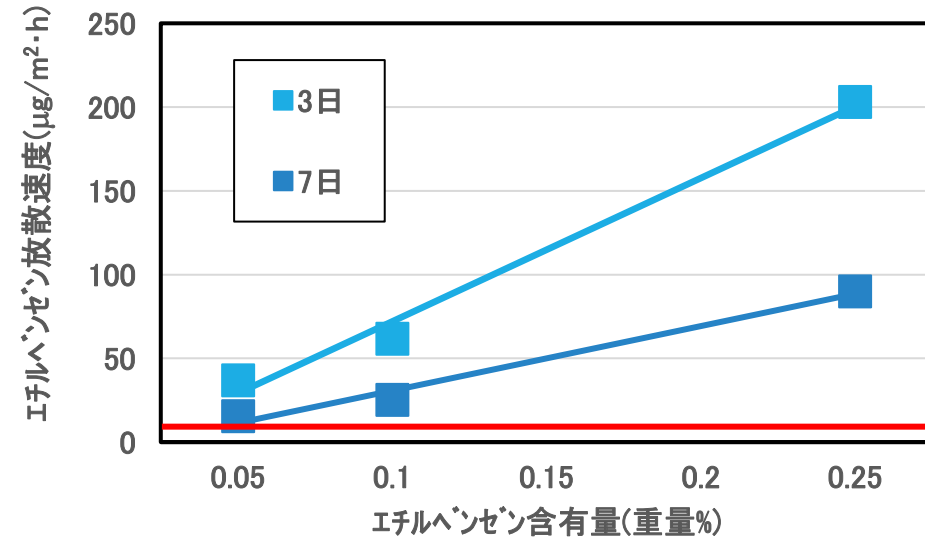
エポキシ樹脂系接着剤のエチルベンゼン放散速度
