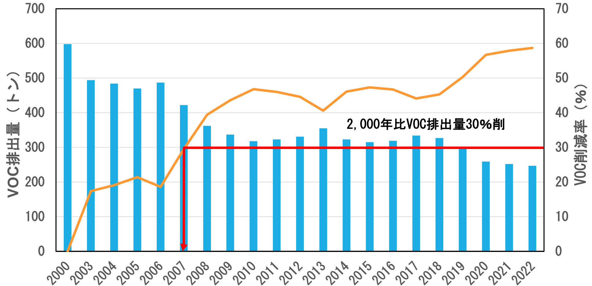
接着剤のVOC排出量推移（9物質）
