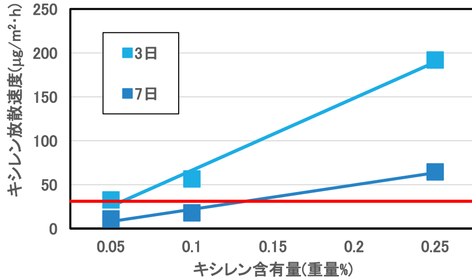
エポキシ樹脂系接着剤のキシレン放散速度
